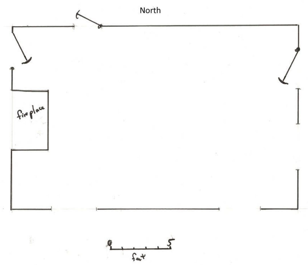
Floor Plan of the LeMeilleur Gallery
